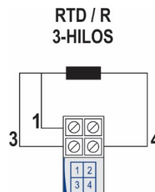
Fig. 8 – Conexiones eléctricas del transmisor (Pt100/Pt1000 3 hilos)
