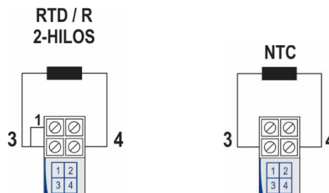
Fig. 7 – Conexiones eléctricas del transmisor (Pt100/Pt1000 2 hilos / NTC)
