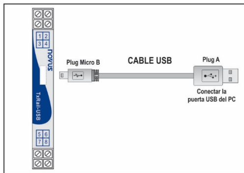
Fig. 1 – Conexión del cable USB
