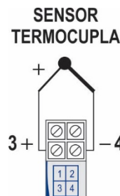
Fig. 10 – Conexiones eléctricas del transmisor (Termocupla)
