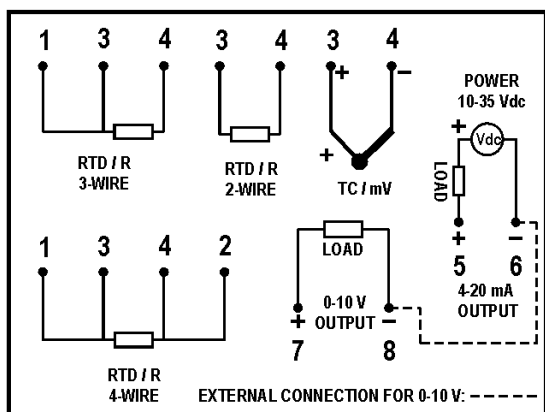
Fig. 6 – Conexiones eléctricas del transmisor TxRail-USB
