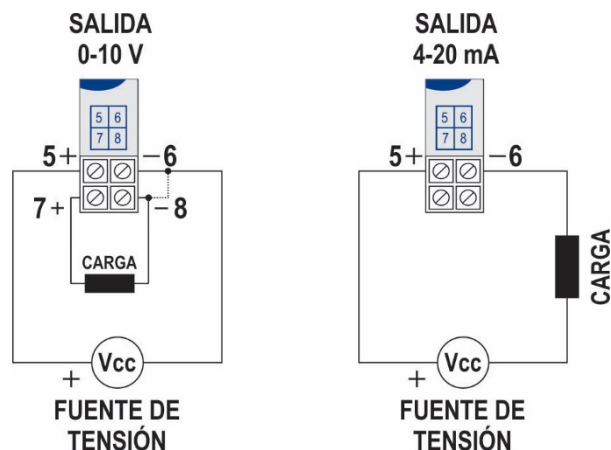
Fig. 12 – Conexiones eléctricas del transmisor (0-10 V y 4-20 mA)
