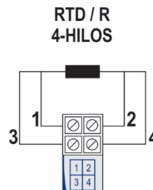
Fig. 9 – Conexiones eléctricas del transmisor (Pt100 4 hilos)
